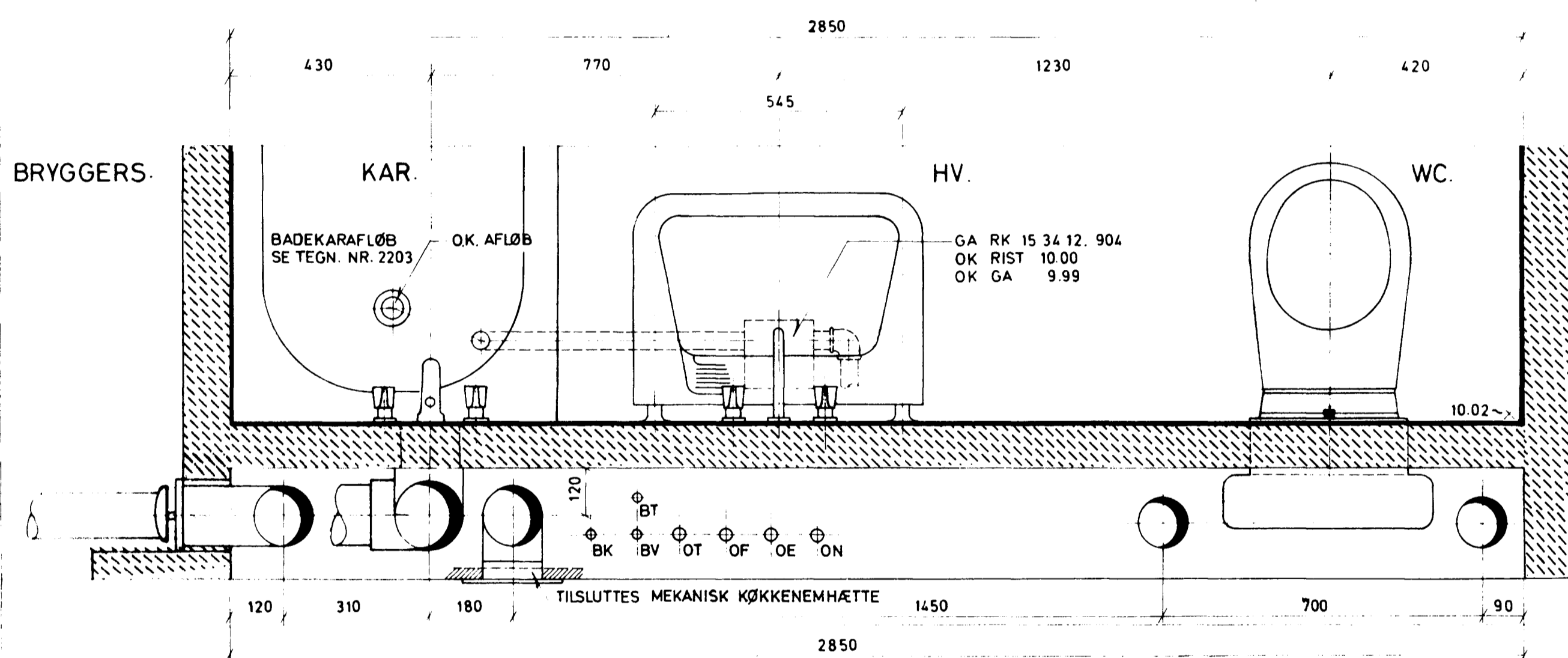
SNIT B-B, PLAN - MELLEMETAGE.
